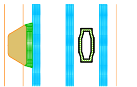
Aussen geklebt mit Zwischenglassprosse
